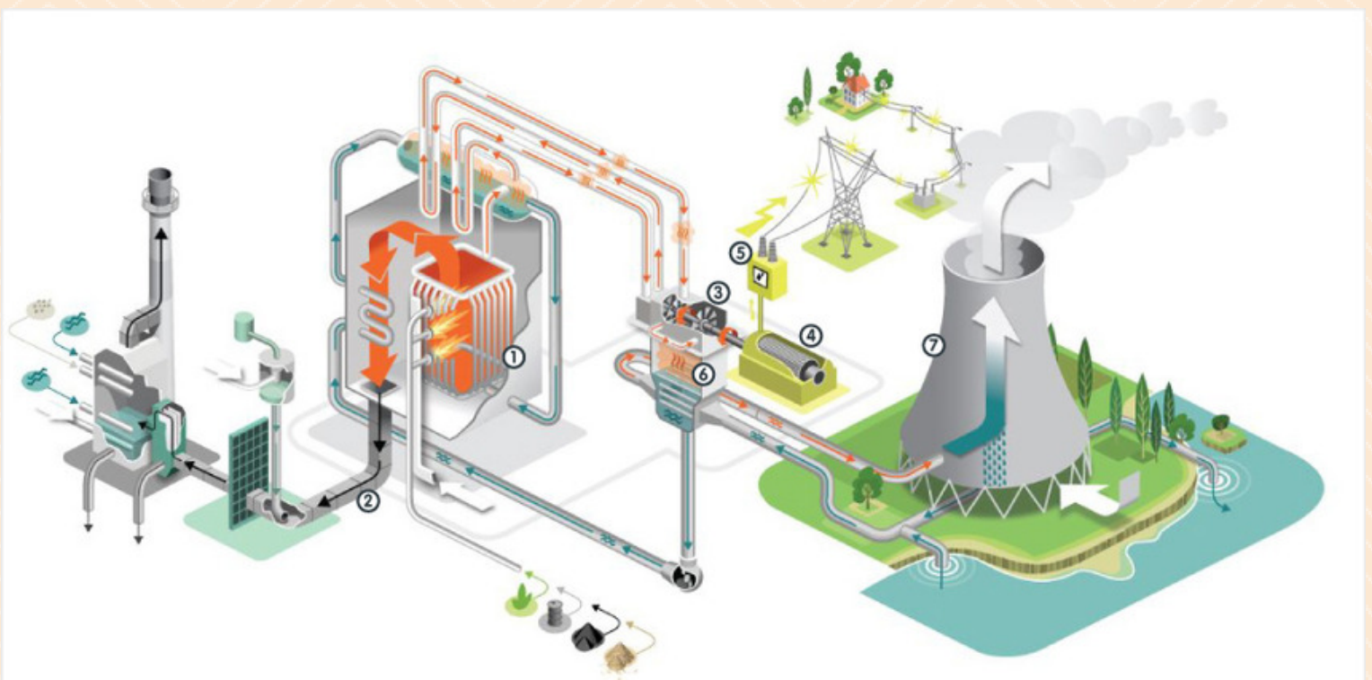
① Chaudière à vapeur ② Électrophiltre ③ Turbine à vapeur ④ Alternateur ⑤ Transformateur ⑥ Condenseur ⑦ Tour de refroidissement
